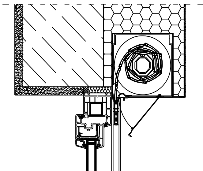
Montaż na ocieplonym nadprożu
