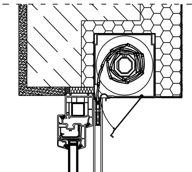
Montaż na „cofniętym nadprożu”
