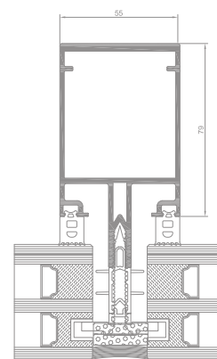
przekrój przez słup systemu MC GLASS
